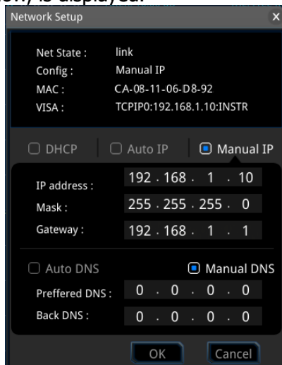
Figure 6-1 LAN Parameter Setting
