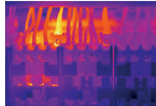
Údržba zařízení: rozpoznání příliš vysokých teplot na pojistkách a elektrických součástkách dříve, než dojde k výpadkům.
